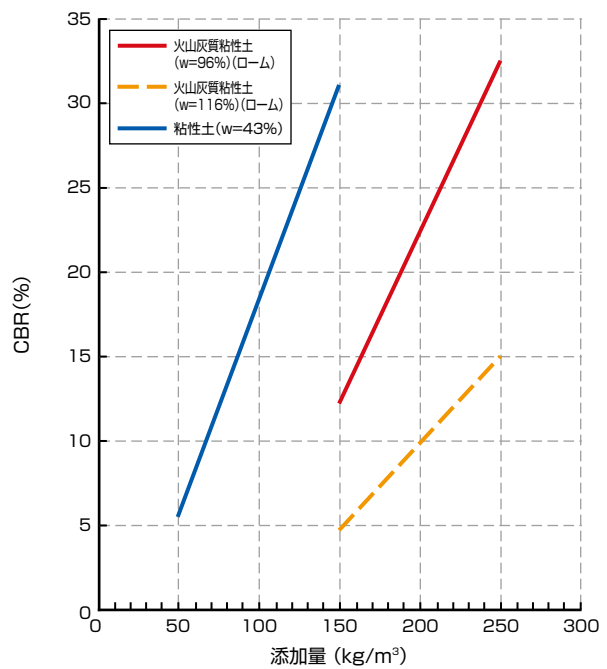
■CBR [材齢7日]
