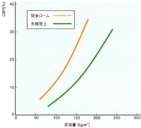
【CBR試験】
