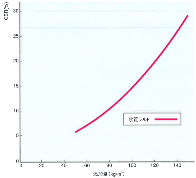
【CBR試験 [ウエットライム]】
