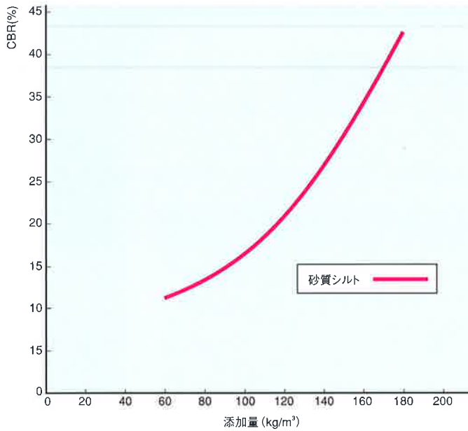
【CBR試験 [消石灰]】
