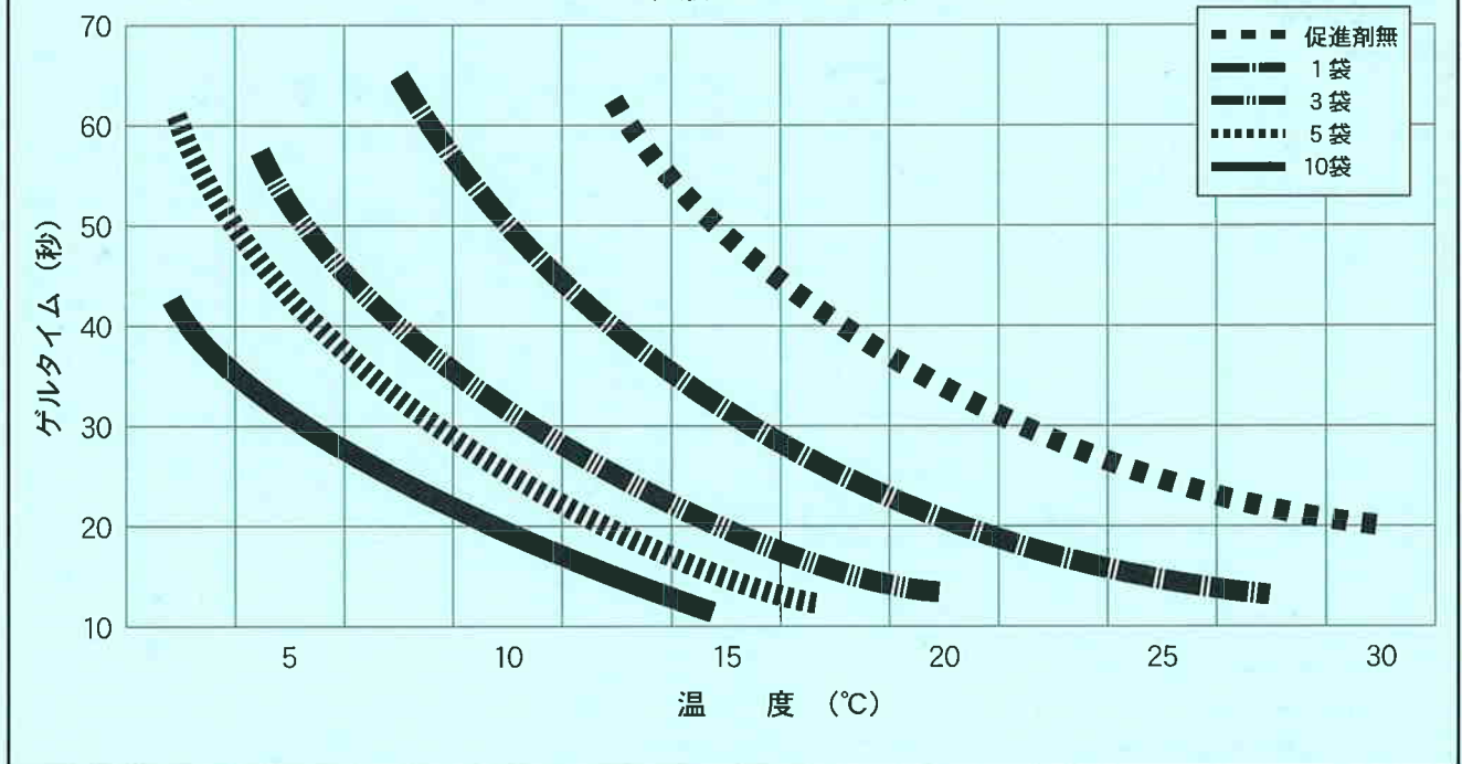
アロンメンダーIIの促進剤量とゲルタイムの関係 (B液33.5ℓ当たり)
